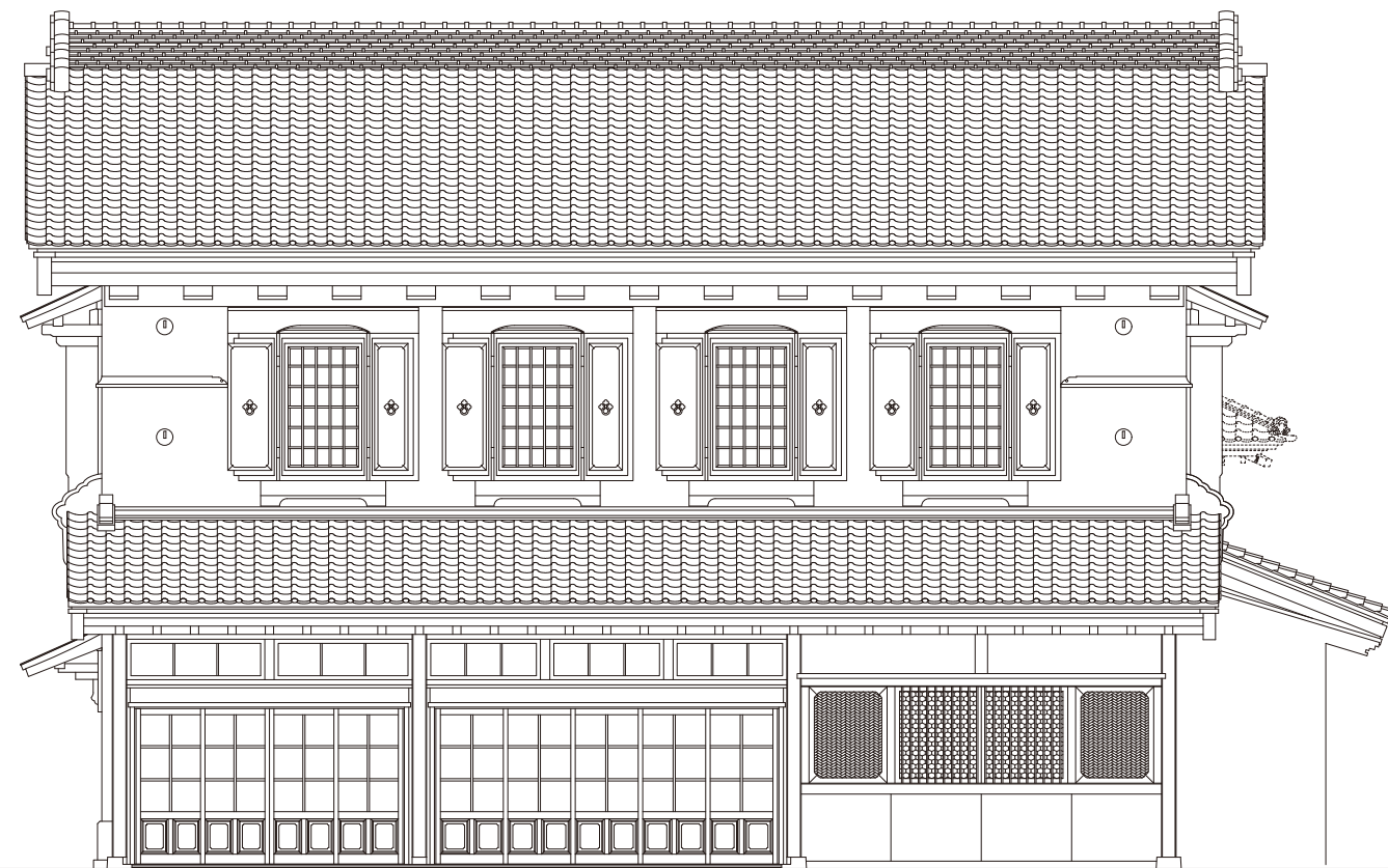
旧甲斐家蔵住宅 店蔵 東側立面図
